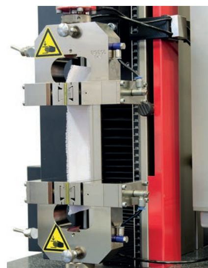
Fig. 2. Tensile test
