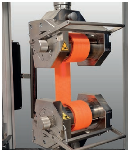
Fig. 3. Roller grips
