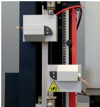
Fig. 2. Capstan grips
